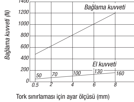
Döner bağlama elemanı 04366-...4540
