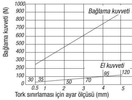
Çekici bağlama elemanı 04400-3240...
