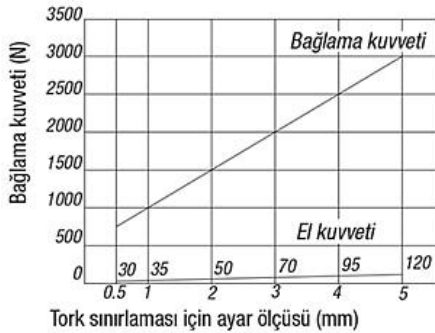
Aşağı çekişli bağlama elemanı 04565-0500 04565-0501
