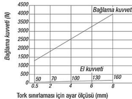
Aşağı çekişli bağlama elemanı 04565-0800 04565-0801
