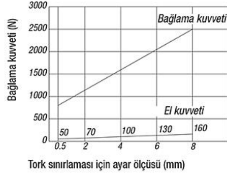
Çekici bağlama elemanı 04400-4050...
