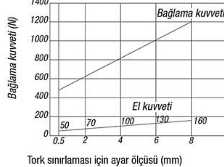
Döner bağlama elemanı 04366-...4540
