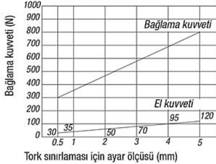
Döner bağlama elemanı 04366-...3232
