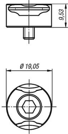
Sıkıştırma tırnağı
