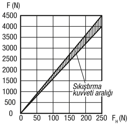
Kuvvet diyagramı
